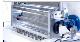
Particolare sistema di taglio trasversale
